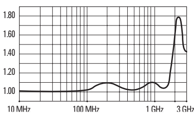
VSWR
